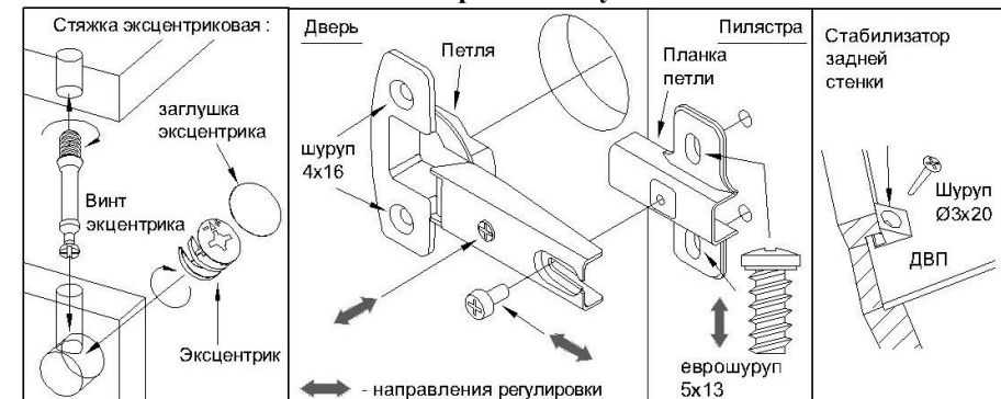
Схема основных крепежных узлов
